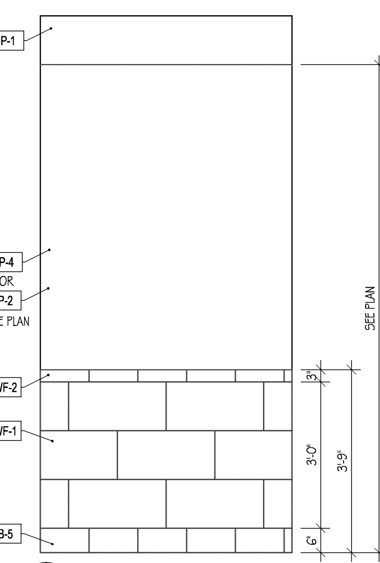
C1 WALL TILE DETAIL @ DINING Scale: N.T.S.
