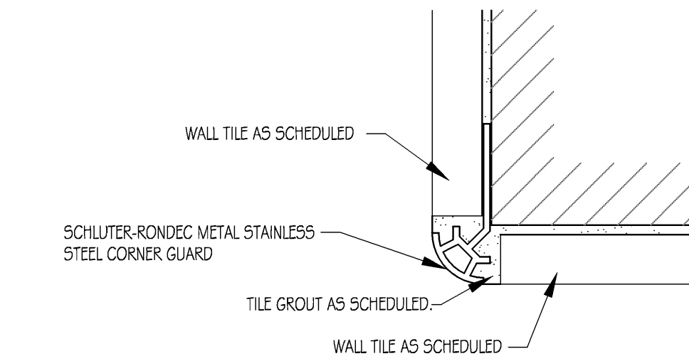
B3 TYPICAL TILE CORNER DETAIL Scale: N.T.S.
