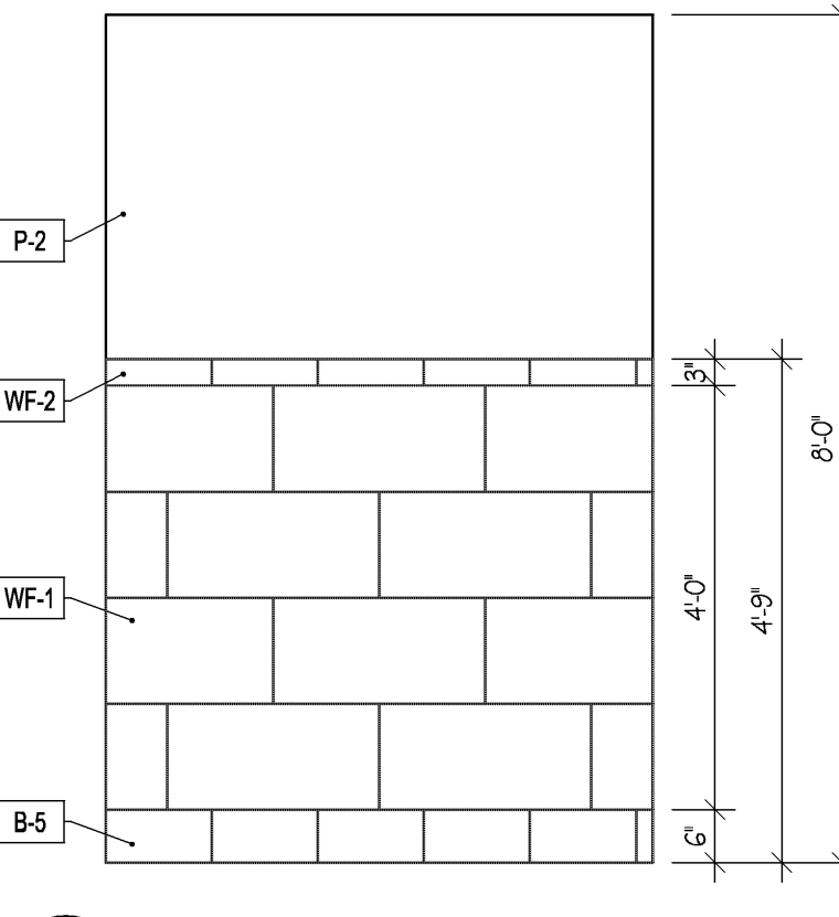
C2 WALL TILE DETAIL @ RESTROOMS Scale: N.T.S.
