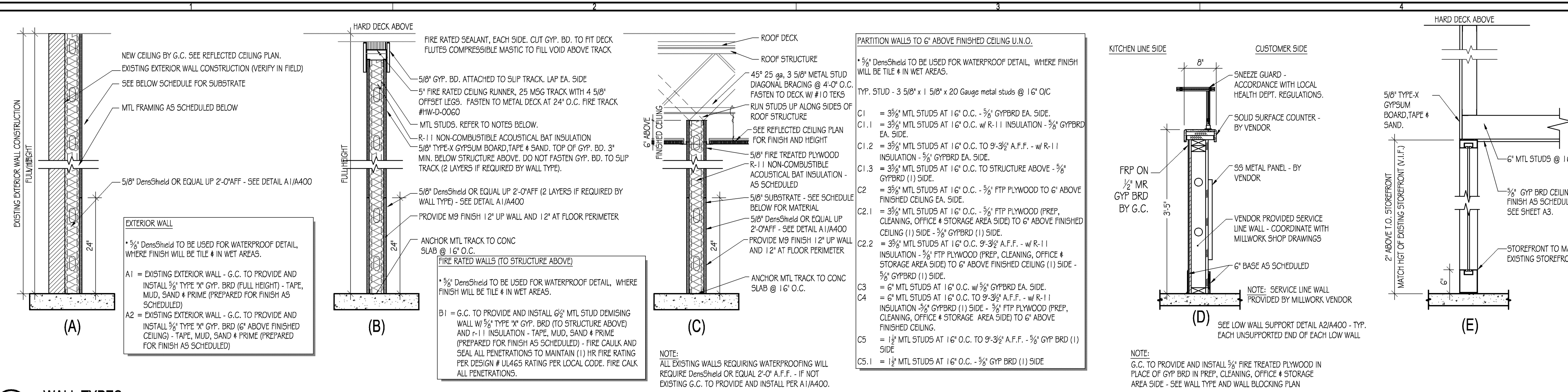
D1 WALL TYPES
